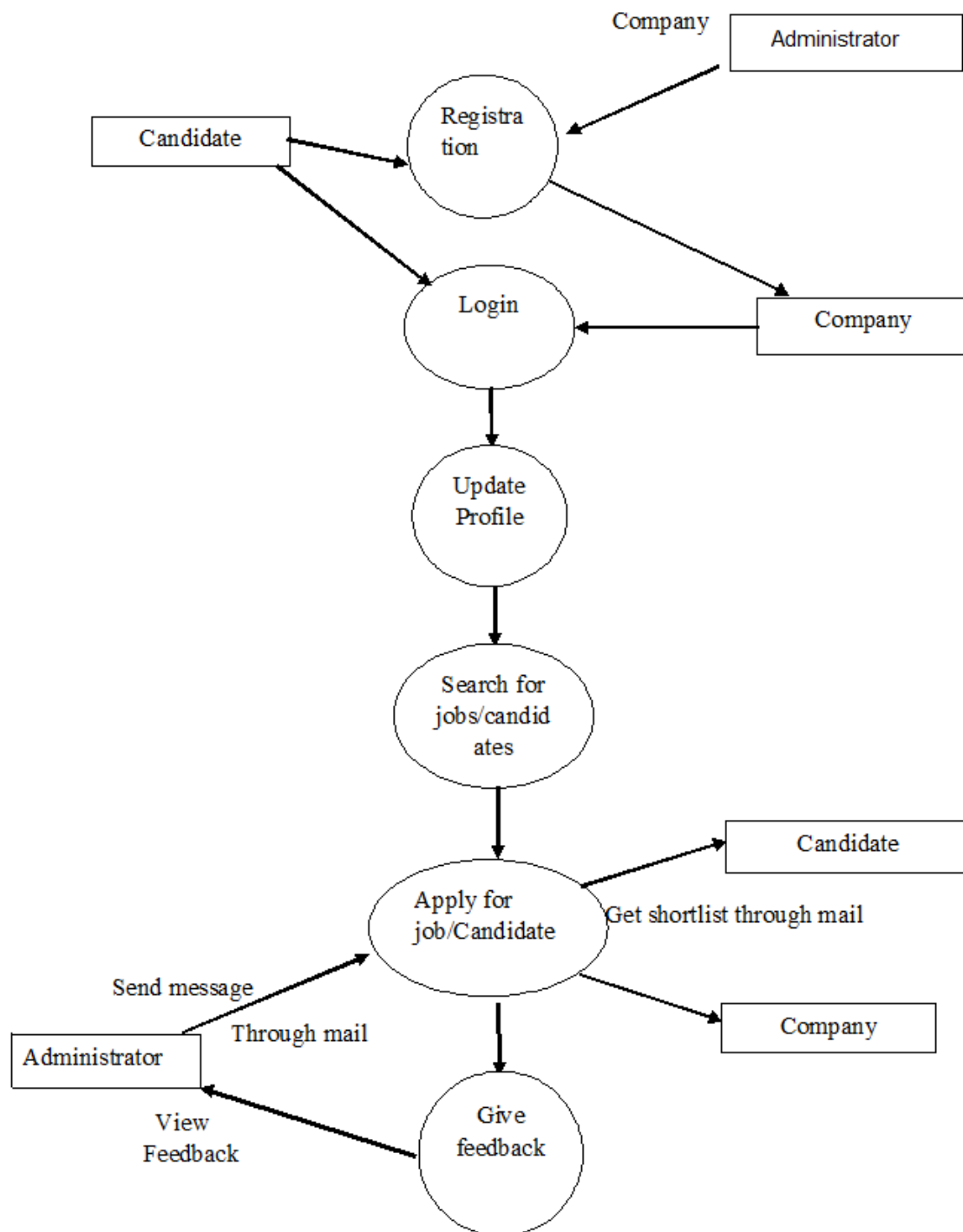
Fig 6.6 : DFD level 2
