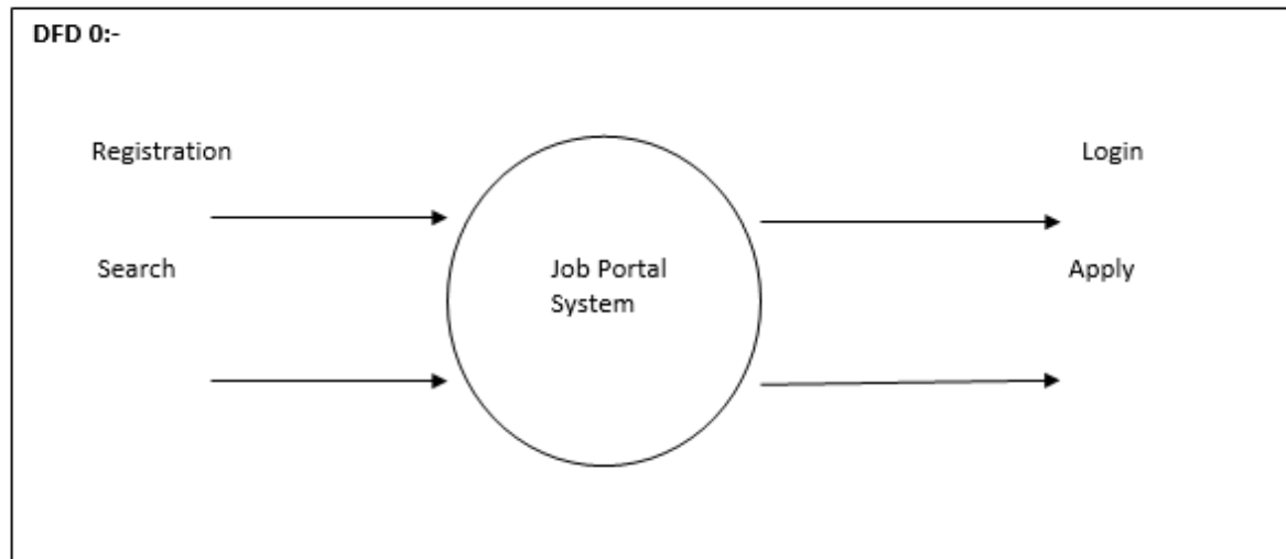
Fig 6.6 : DFD level 0
