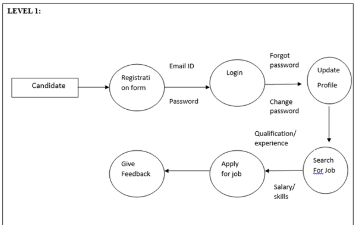
Fig 6.6 : DFD level 1
